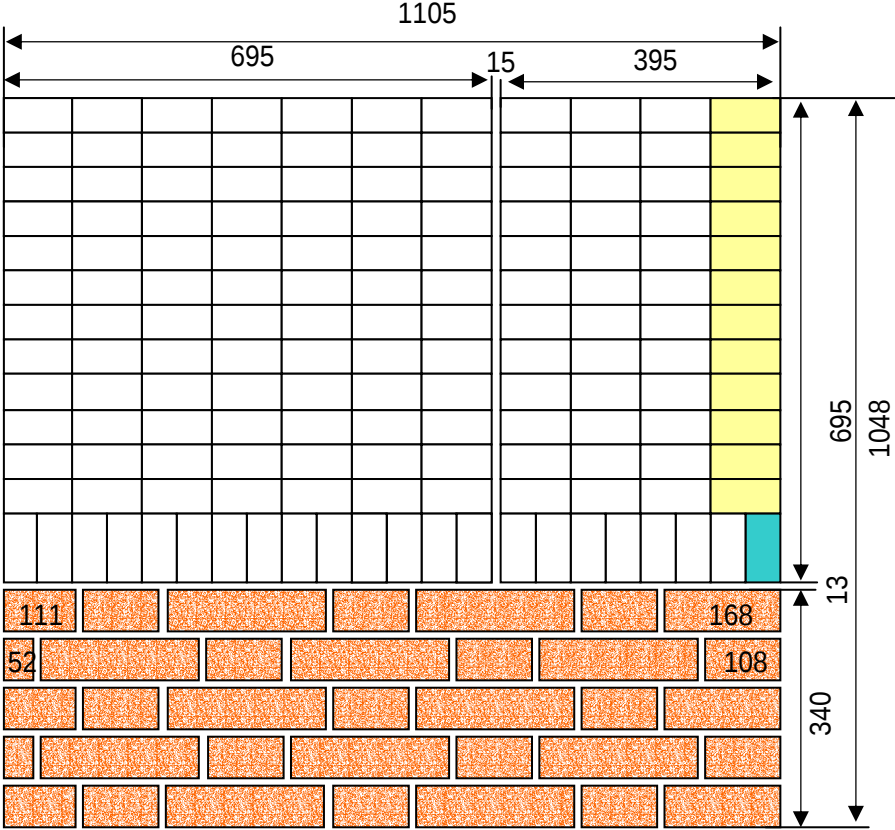
製作図
